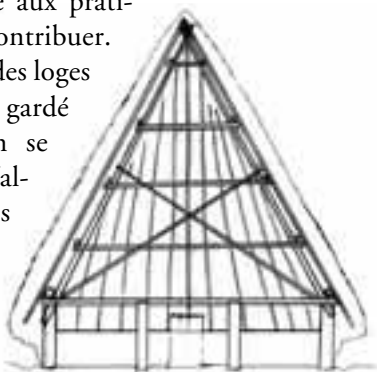
Coupe de la loge du Haut-Davy, dessin Gérard Baptiste.
